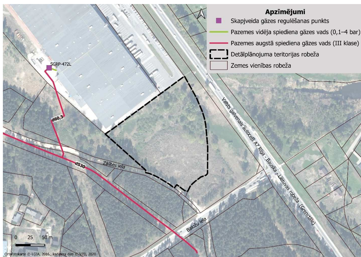
26. attēls. Gāzapgādes tīkli un objekti
